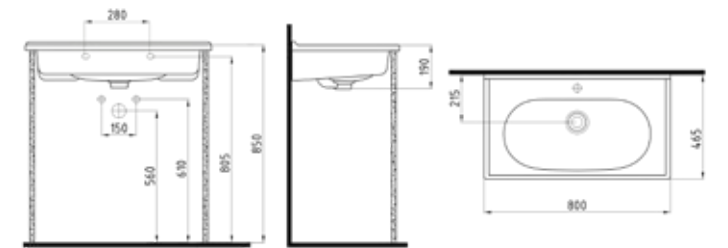
KONSOLLU LAVABO BATARYA DELİKLİ / TAŞMA DELİKLİ FELK080B1FD1W5000 800x465 mm Beyaz
