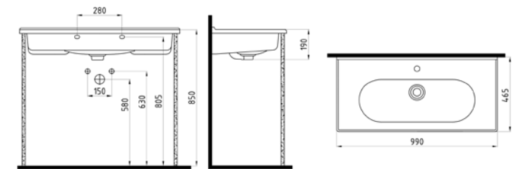
KONSOLLU LAVABO BATARYA DELİKLİ / TAŞMA DELİKLİ FELK100B1FD1W5000 1000x465 mm Beyaz
