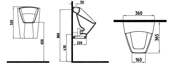
PİSUAR NPPS05201VSAW5000 (Arkadan Su Girişli) 520x365 mm
