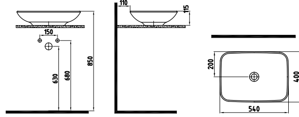
GÖVDE ÜSTÜ DİKDÖRTGEN LAVABO BATARYA DELİKSİZ TAŞMA DELİKSİZ HRLG05401FDOW5000 540x400 mm
