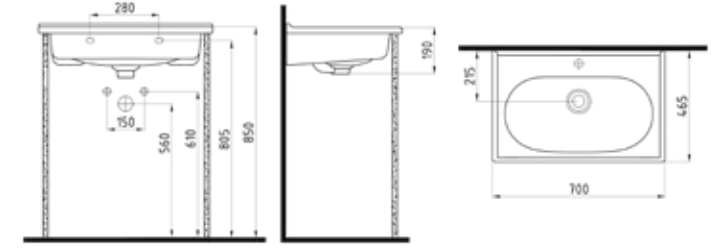
KONSOLLU LAVABO BATARYA DELİKLİ / TAŞMA DELİKLİ FELK070B1FD1W5000 700x465 mm Beyaz
