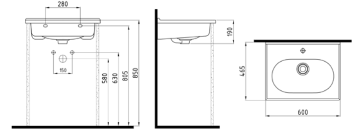
KONSOLLU LAVABO BATARYA DELİKLİ / TAŞMA DELİKLİ FELK060B1FD1W5000 600x465 mm Beyaz
