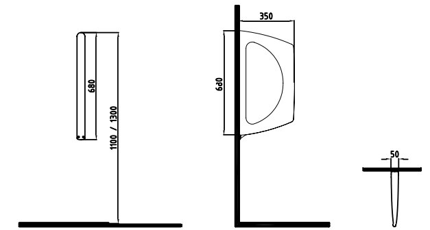
PİSUAR ARA BÖLME NPPA06801V00W5000 680x350 mm
