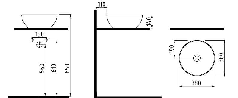
GÖVDE ÜSTÜ LAVABO BATARYA DELİKSİZ / TAŞMA DELİKSİZ MTLG03802FD0W5000 Ø 380 mm
